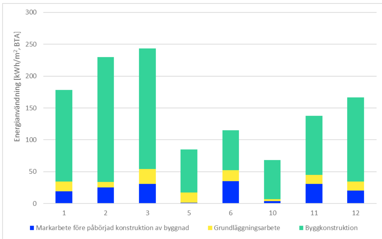
Figur 31 Energianvändning per kvadratmeter fördelad per byggfas för de åtta projekten som inkluderat markarbetet före påbörjad konstruktion av byggnad. Y-axeln visar energianvändningen i kWh/m², BTA och X-axeln visar byggprojekt ID.
