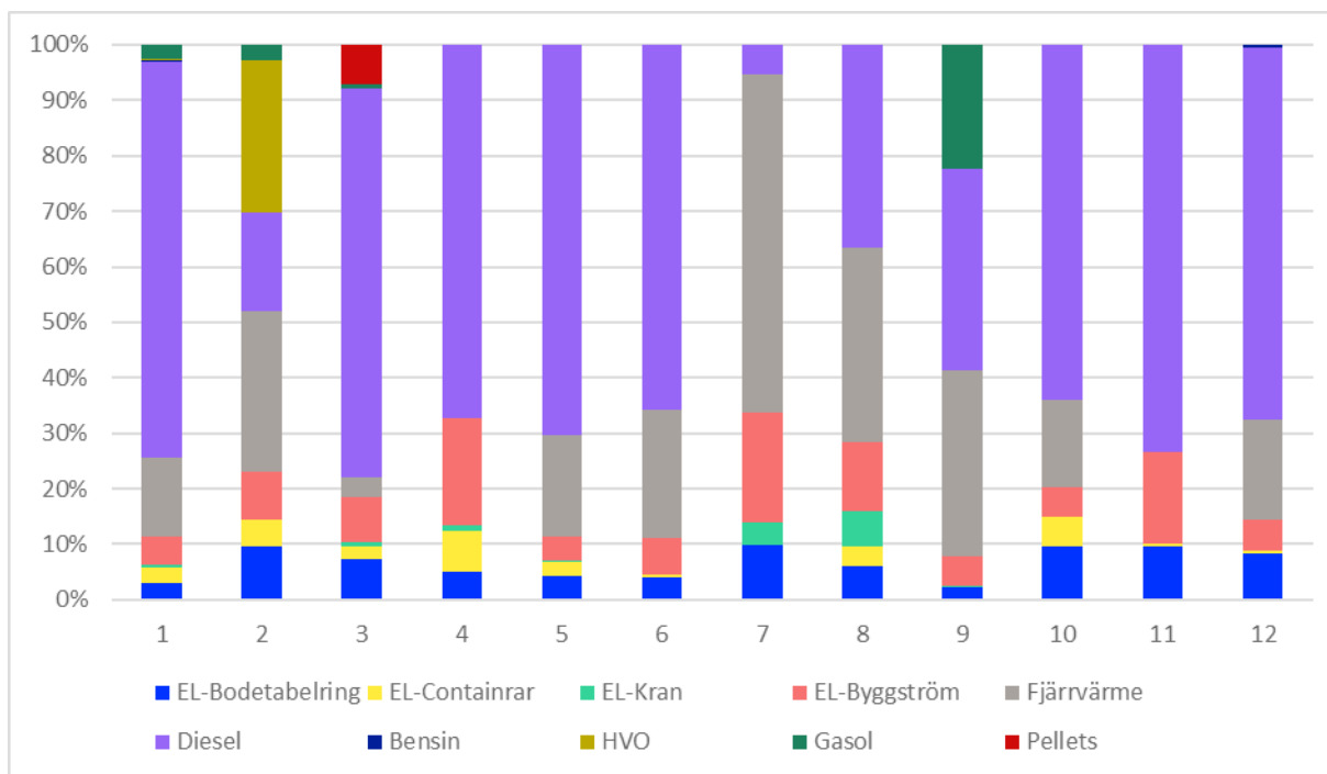
Figur 41 Fördelning mellan olika energislag och aktivitet för de 12 byggprojekten. X-axeln visar byggprojekt ID.
