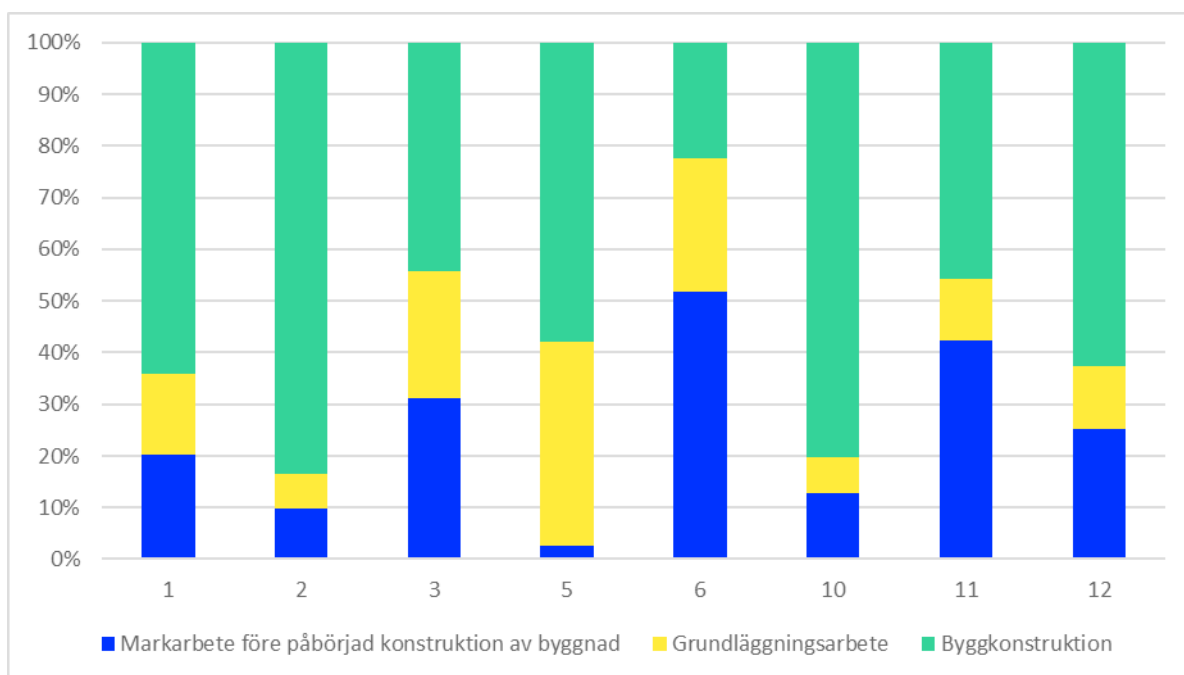
Figur 43 Fördelning mellan byggfaser för de åtta projekten som inkluderat markarbetet före påbörjad konstruktion av byggnad. X-axeln visar byggprojekt ID.
