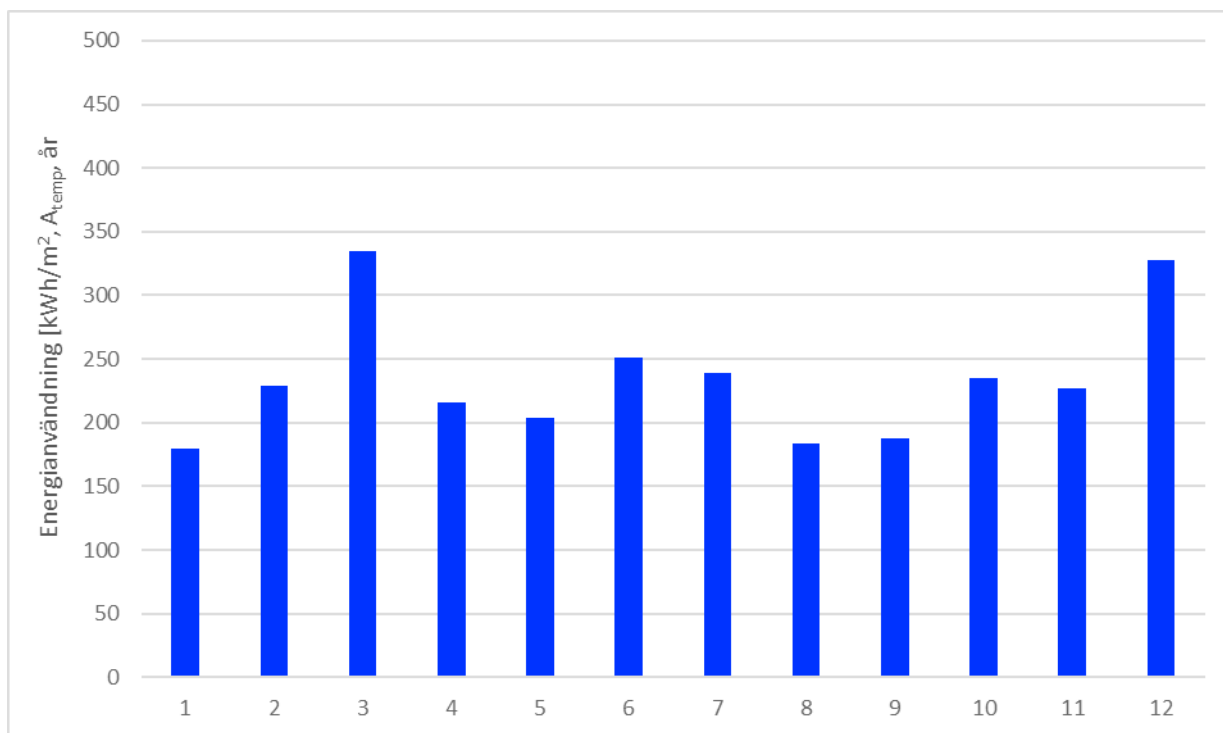
Figur 16 Årlig energianvändning per kvadratmeter A_{temp} för projekten. Y-axeln visar energianvändning i kWh/m 2 , A_{temp} , år och X-axeln visar byggprojekt ID.
