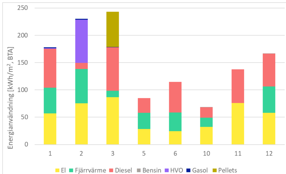
Figur 11 Energianvändning per kvadratmeter uppdelat per energislag inklusive energianvändning för markarbete före påbörjad konstruktion av byggnad. Y-axeln visar energianvändningen i kWh/m², BTA och X-axeln visar byggprojekt ID.
