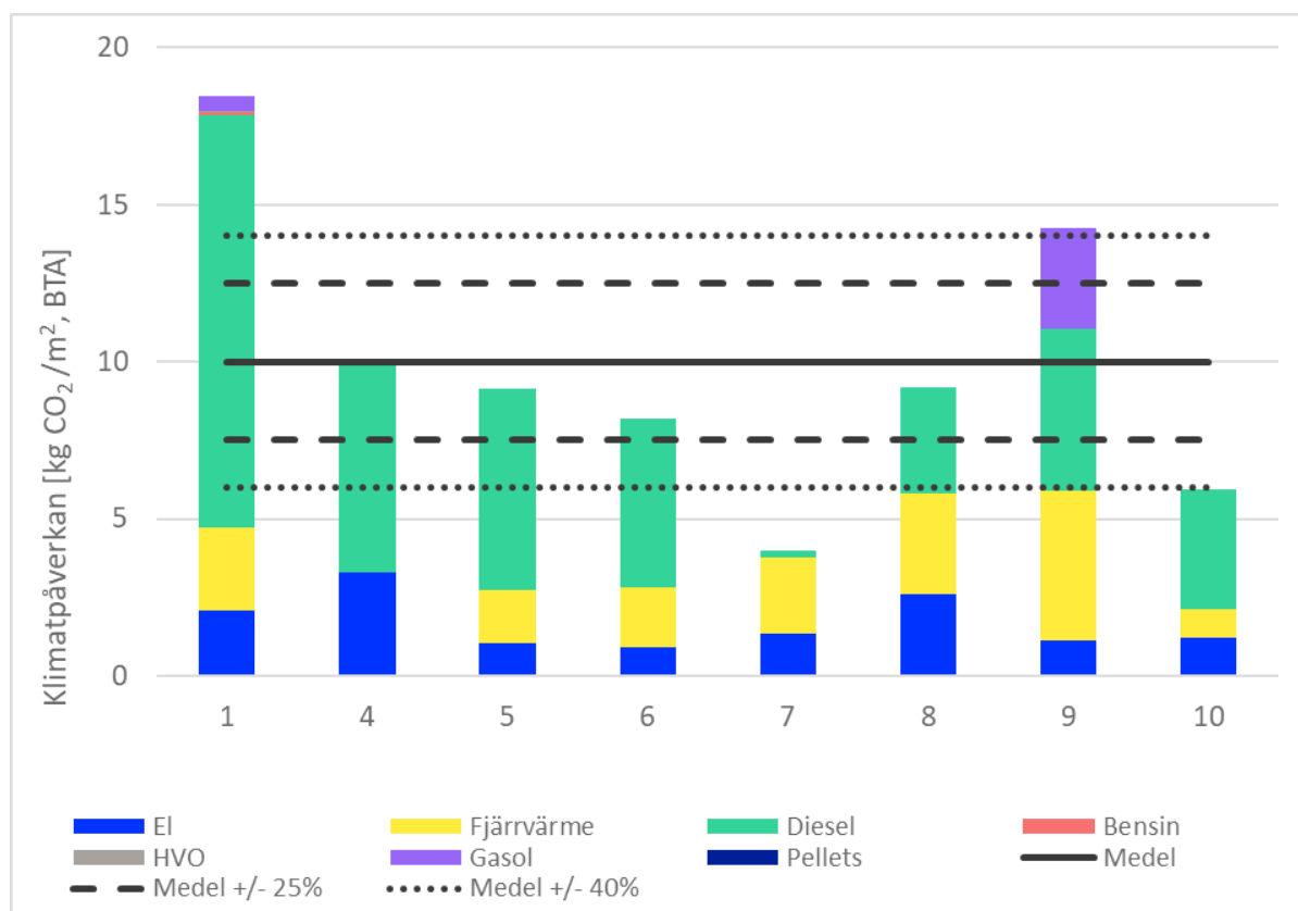
Figur 37 Klimatpåverkan per kvadratmeter och medelvärde för flerbostadshusprojekten inklusive procentuella avvikelser från medelvärdet. Y-axeln visar klimatpåverkan i kg CO 2 -ekv/m 2 , BTA och X-axeln visar byggprojekt ID.
