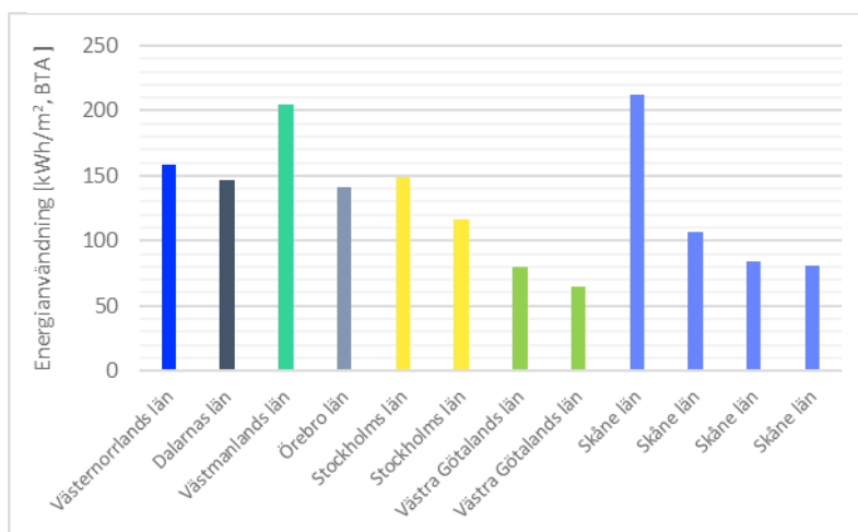
Figur 12 Årlig energianvändning per kvm byggprojekten och respektive län som de uppförts i. Y-axeln visar energianvändningen i kWh/m², BTA, år och X-axeln visar län i Sverige
