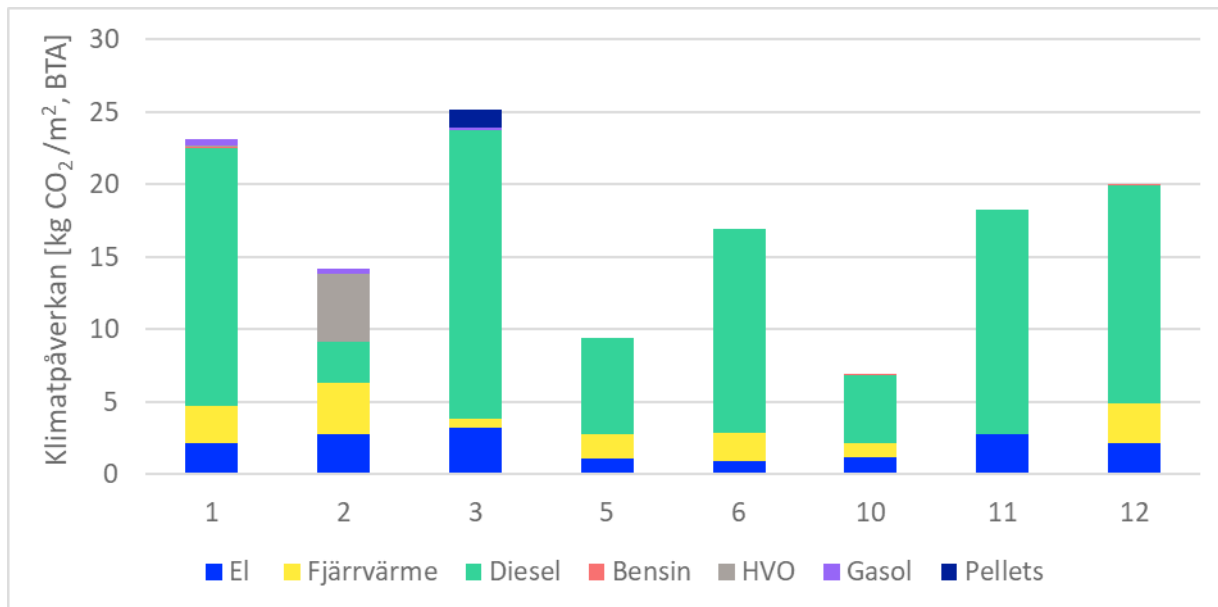
Figur 39 Klimatpåverkan per kvadratmeter uppdelat per energislag inklusive klimatpåverkan från energianvändning för markarbete före påbörjad konstruktion av byggnad. Y-axeln visar klimatpåverkan i kg CO 2 -ekv/m 2 , BTA och X-axeln visar byggprojekt ID.
