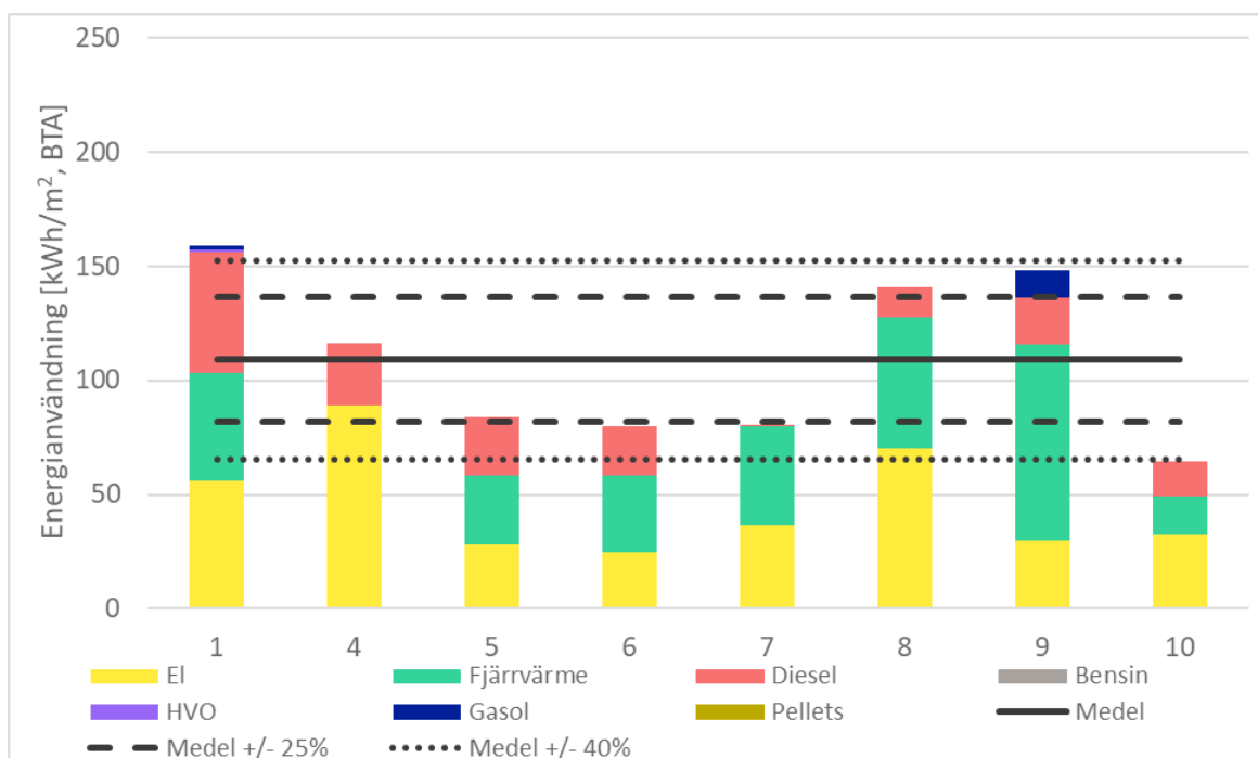
Figur 5 Energianvändning per kvadratmeter och medelvärde för flerbostadshusprojekten inklusive procentuella avvikelser från medelvärdet. Y-axeln visar energianvändningen i kWh/m², BTA och X-axeln visar byggprojekt ID.
