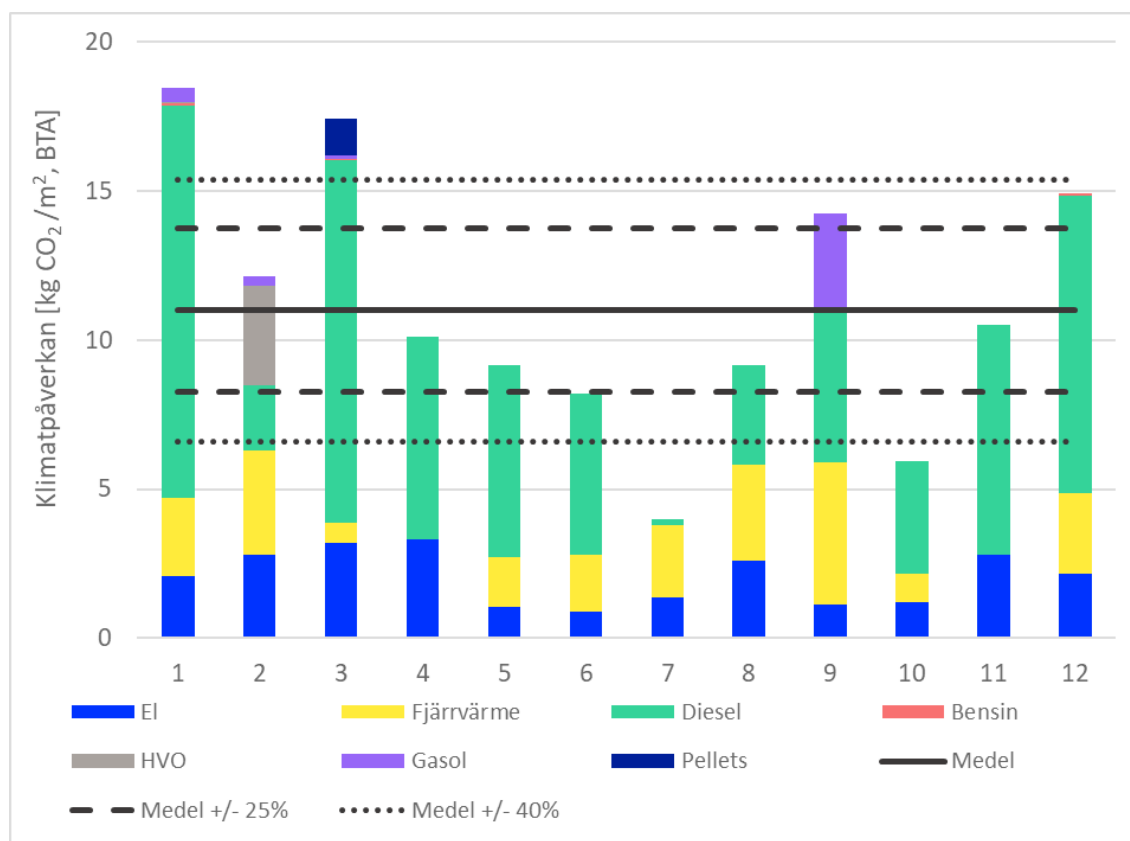
Figur 36 Klimatpåverkan per kvadratmeter och medelvärde för de 12 projekten inklusive procentuella avvikelser från medelvärdet. Y-axeln visar klimatpåverkan i kg CO 2 -ekv/m 2 , BTA och X-axeln visar byggprojekt ID.
