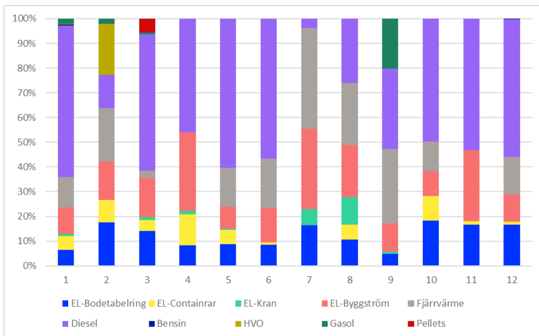
Figur 45 Klimatpåverkan. Fördelning mellan olika energislag för de 12 byggprojekten beräknat med nordisk elmix. X-axeln visar byggprojekt ID.
