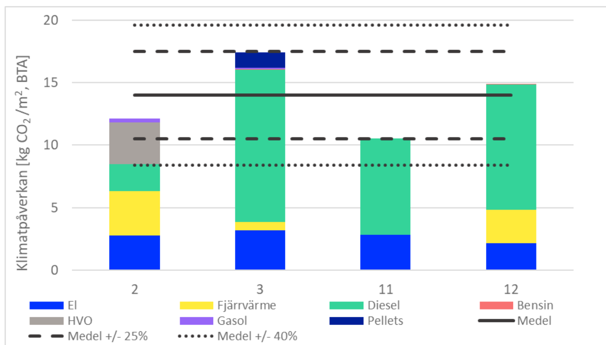
Figur 38 Klimatpåverkan per kvadratmeter och medelvärde för de projekt där skolor/större förskolor byggdes inklusive procentuella avvikelser från medelvärdet. Y-axeln visar klimatpåverkan i kg CO 2 -ekv/m 2 , BTA och X-axeln visar byggprojekt ID.
