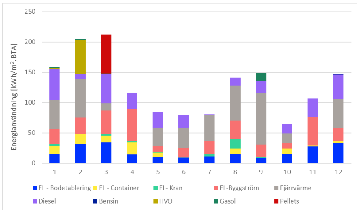
Figur 29 Energianvändning per kvadratmeter uppdelat per energislag och aktivitet. Y-axeln visar energianvändningen i kWh/m², BTA och X-axeln visar byggprojekt ID.
