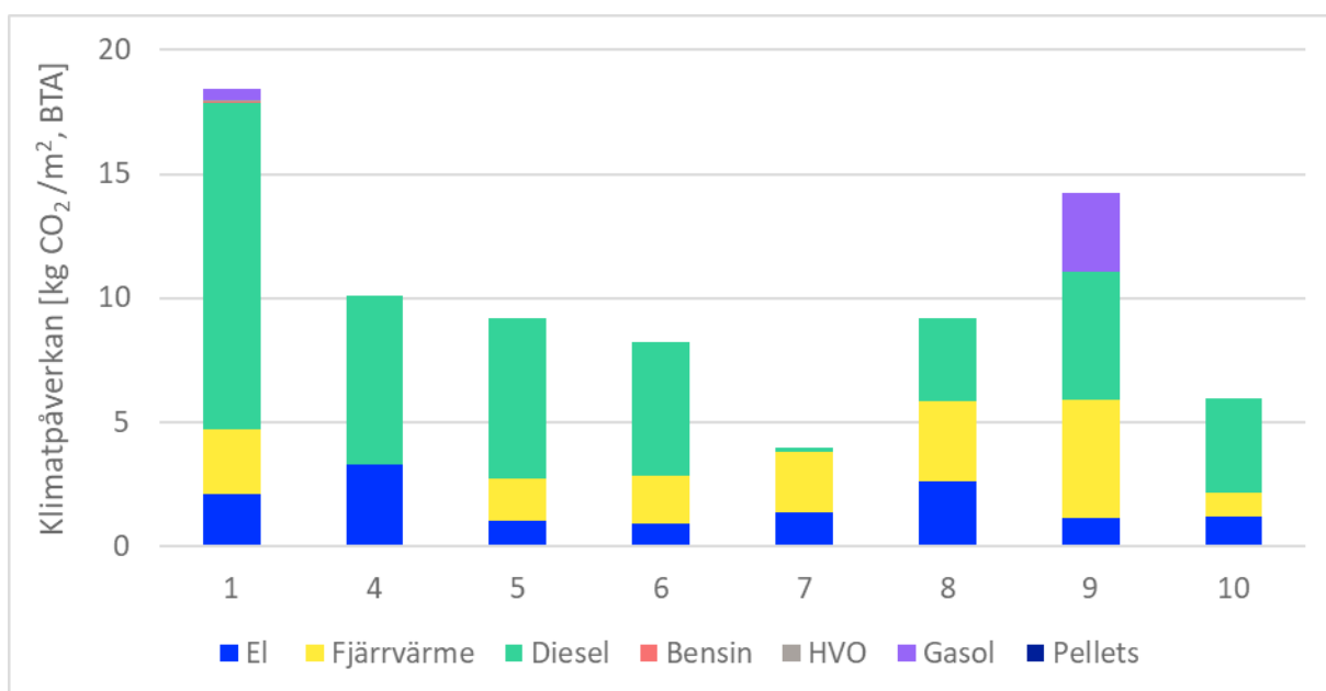
Figur 34 Klimatpåverkan uppdelat per energislag för flerbostadshusprojekten. Y-axeln visar klimatpåverkan i kg CO 2 -ekv/m 2 , BTA och X-axeln visar byggprojekt ID.
