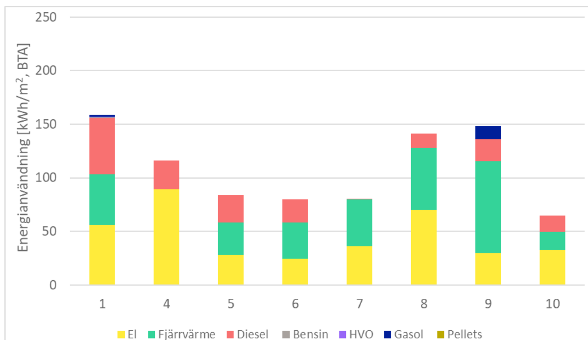
Figur 2 visar energianvändningen per kvadratmeter uppdelat per energislag för de 8 flerbostadshusprojekten. Energianvändningen ligger mellan 65 och 159 kWh/m 2 , BTA.
