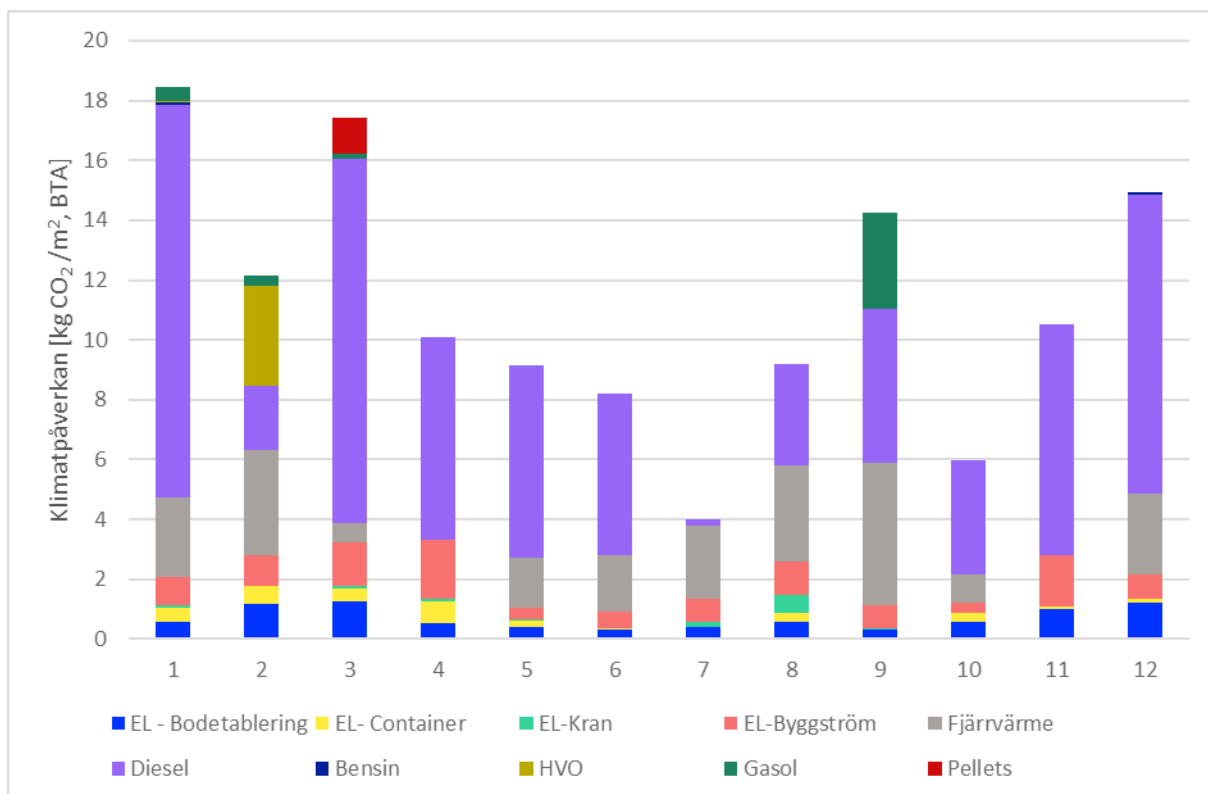
Figur 40 Klimatpåverkan per kvadratmeter uppdelat per energislag och aktivitet. Y-axeln visar klimatpåverkan i kg CO 2 -ekv/m 2 , BTA och X-axeln visar byggprojekt ID.
