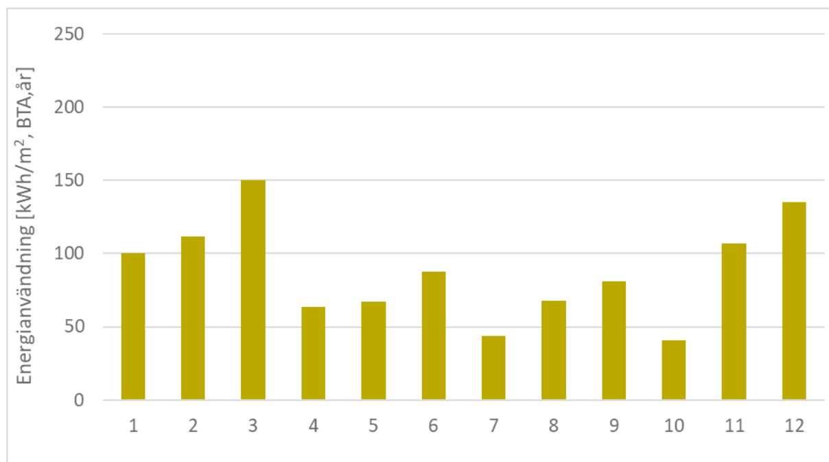
Figur 7 Årlig energianvändningen per kvadratmeter. Y-axeln visar energianvändningen i kWh/m 2 , BTA och år och X-axeln visar byggprojekt ID.
