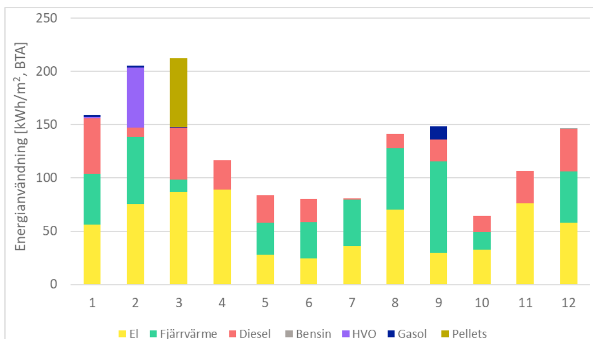
Figur 1 Energianvändning per kvadratmeter uppdelat per energislag. Y-axeln visar energianvändningen i kWh/m 2 , BTA och X-axeln visar byggprojekt ID.
