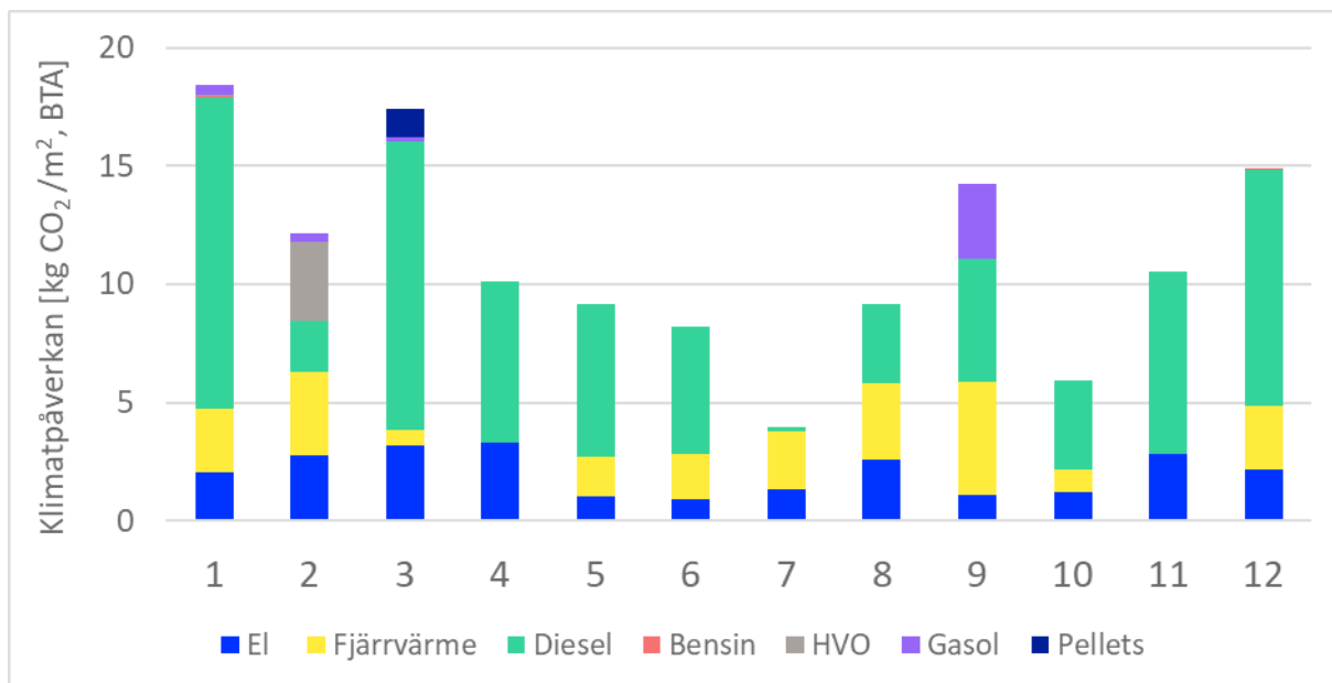
Figur 33 Klimatpåverkan uppdelat per energislag. Y-axeln visar klimatpåverkan i kg CO 2 -ekv/m 2 , BTA och X-axeln visar byggprojekt ID.
