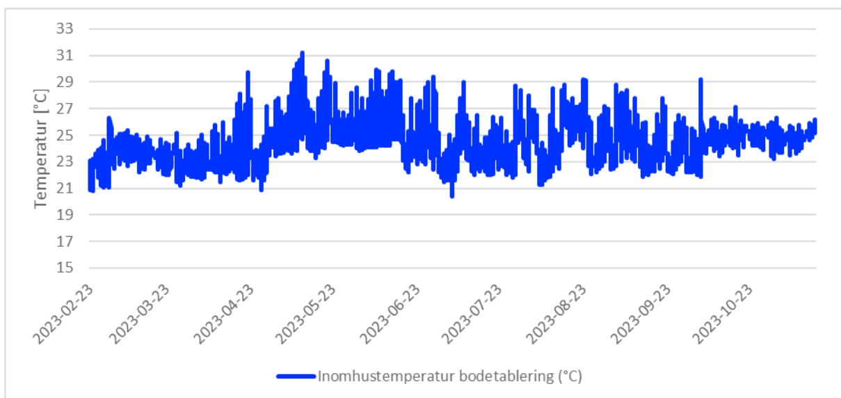
Figur 20 Inomhustemperaturer i bodetableringen från februari-november 2023.
