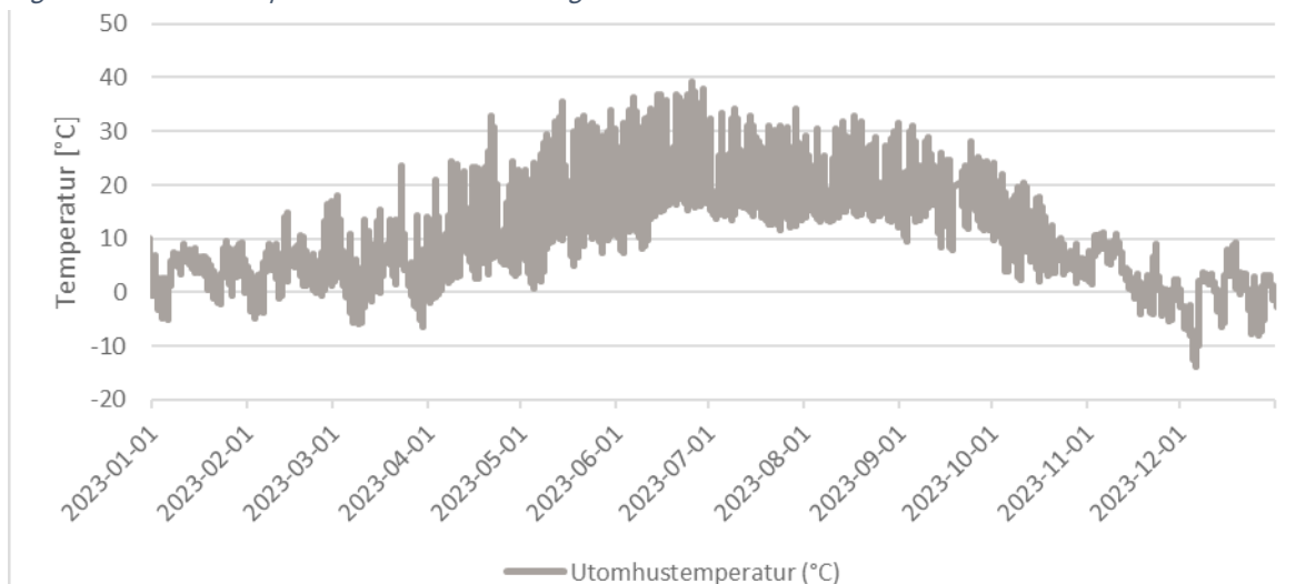
Figur 18 Uppmätt utomhustemperatur
