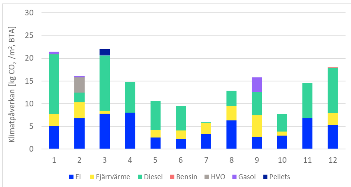
Figur 44 Klimatpåverkan uppdelat per energislag beräknad med nordisk elmix. Y-axeln visar klimatpåverkan i kg CO 2 -ekv/m², BTA och X-axeln visar byggprojekt ID.
