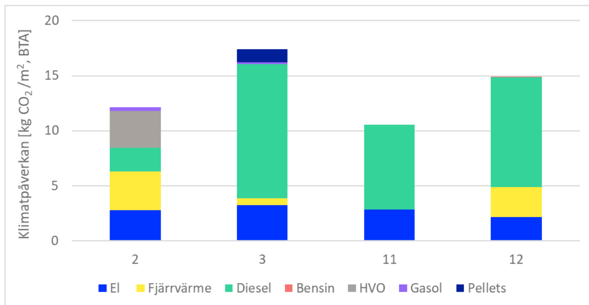
Figur 35 Klimatpåverkan uppdelat per energislag för projekten där skola/större förskola byggdes. Y-axeln visar klimatpåverkan i kg CO 2 -ekv/m 2 , BTA och X-axeln visar byggprojekt ID.
