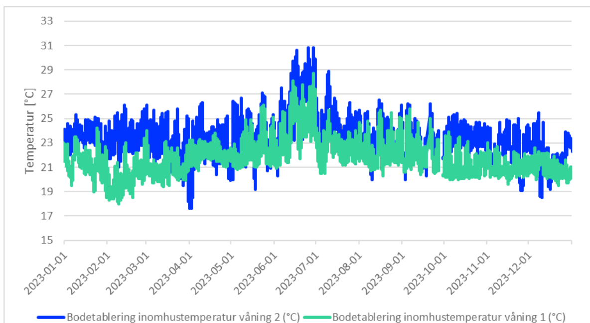
Figur 17 Inomhustemperaturer i bodetableringen under 2023.
