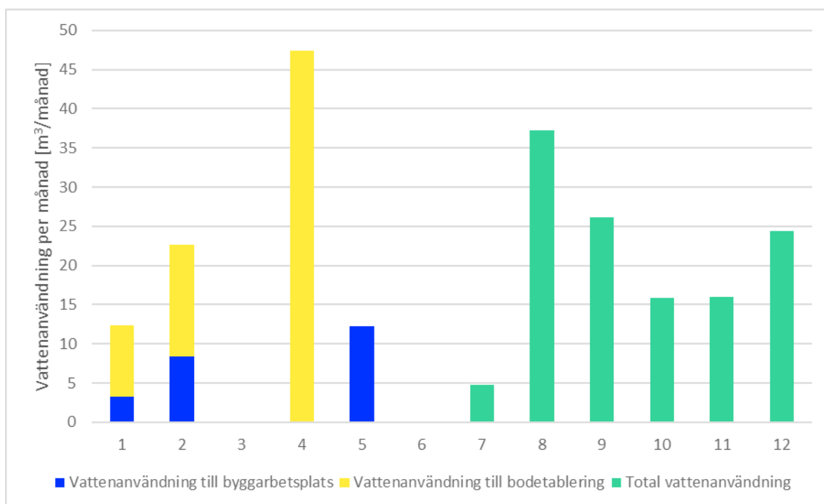
Figur 28 Vattenanvändning per månad för de 12 byggprojekten. Y-axeln visar Vattenanvändning m^3/månad och X-axeln visar byggprojekt ID.
