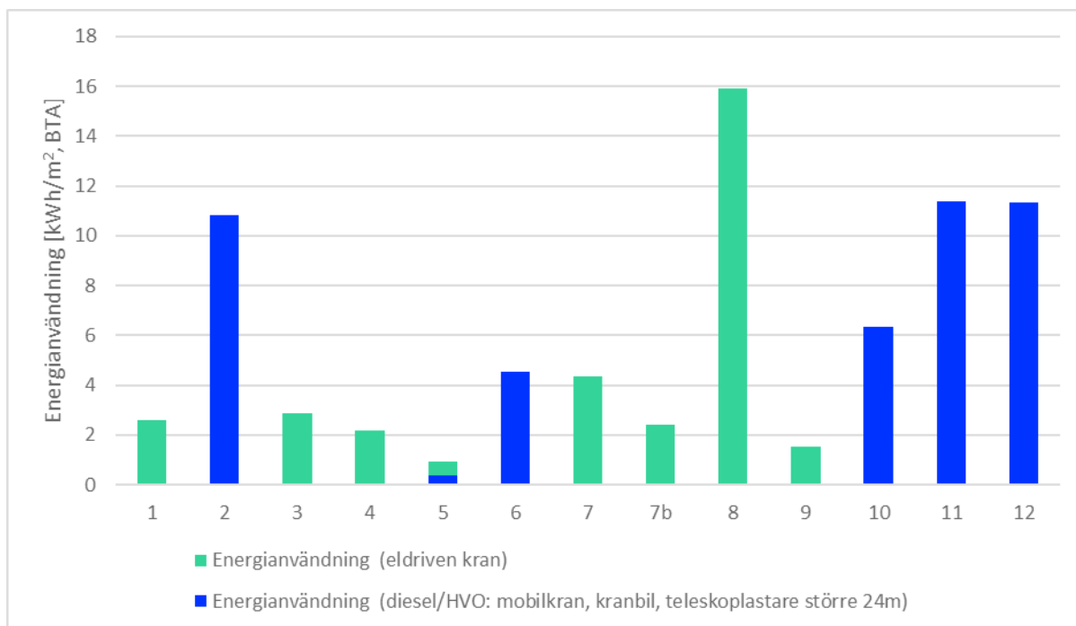
Figur 26 Energianvändning per kvadratmeter BTA för eldrivna kranar samt kranar som drivs med HVO eller diesel (mobilkranar, kranbil, teleskoplastare modell större, över 24 m). Y-axeln visar energianvändningen i kWh/m 2 , BTA och X-axeln visar byggprojekt ID.
