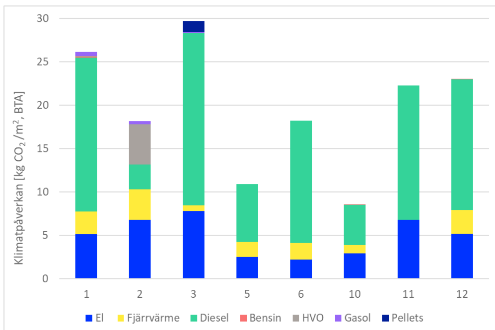
Figur 46 Klimatpåverkan per kvadratmeter uppdelat per energislag inklusive klimatpåverkan från energianvändning för markarbete före påbörjad konstruktion av byggnad. Y-axeln visar klimatpåverkan i kg CO 2 -ekv/m 2 , BTA och X-axeln visar byggprojekt ID.
