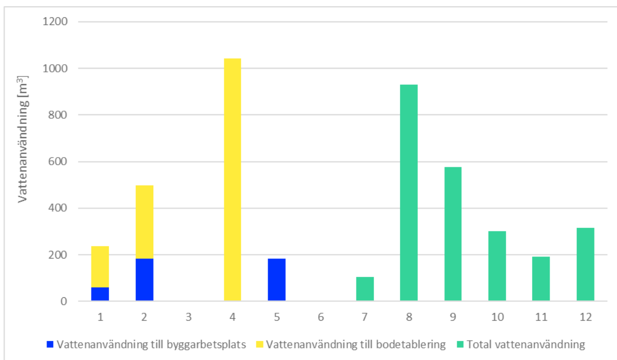
Figur 27 Vattenanvändning för de 12 byggprojekten. Y-axeln visar Vattenanvändning m^3 och X-axeln visar byggprojekt ID.
