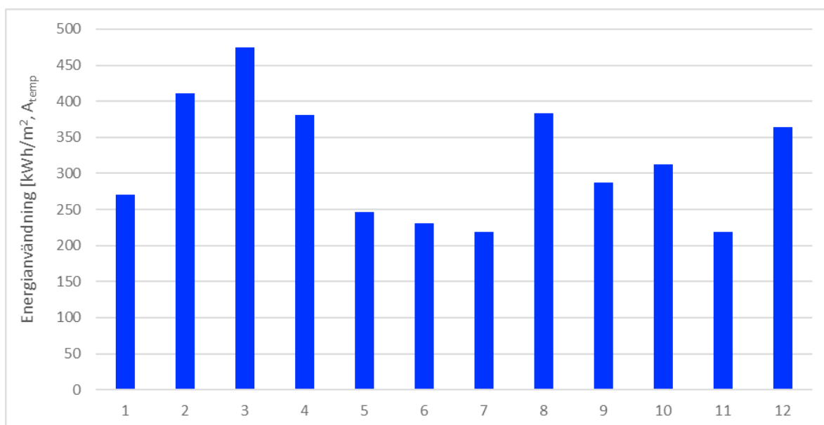
Figur 15 Energianvändning per kvadratmeter A_{temp} för projekten. Y-axeln visar energianvändning i kWh/m 2 , A_{temp} och X-axeln visar byggprojekt ID.
