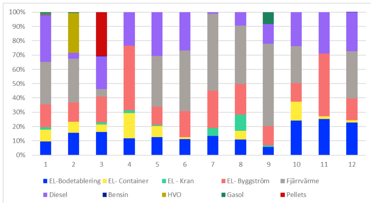
Figur 30 Fördelning mellan olika energislag och aktiviteter för de 12 byggprojekten. X-axeln visar byggprojekt ID.
