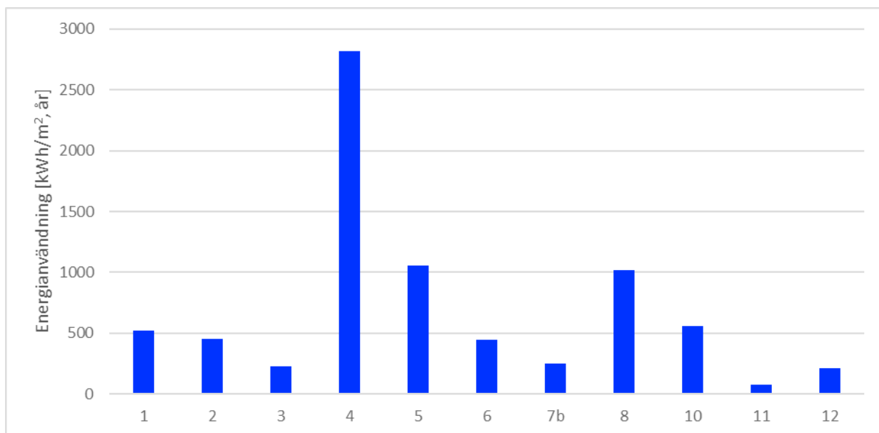
Figur 24 Årlig energianvändning per kvadratmeter. Y-axeln visar energianvändning i kWh/m 2 , år och X-axeln visar byggprojekt ID.
